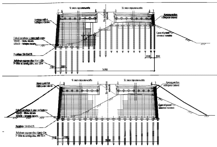
Рис. 8.22. Конструктивные решения для переходных участков на безосадочном свайном основании.
