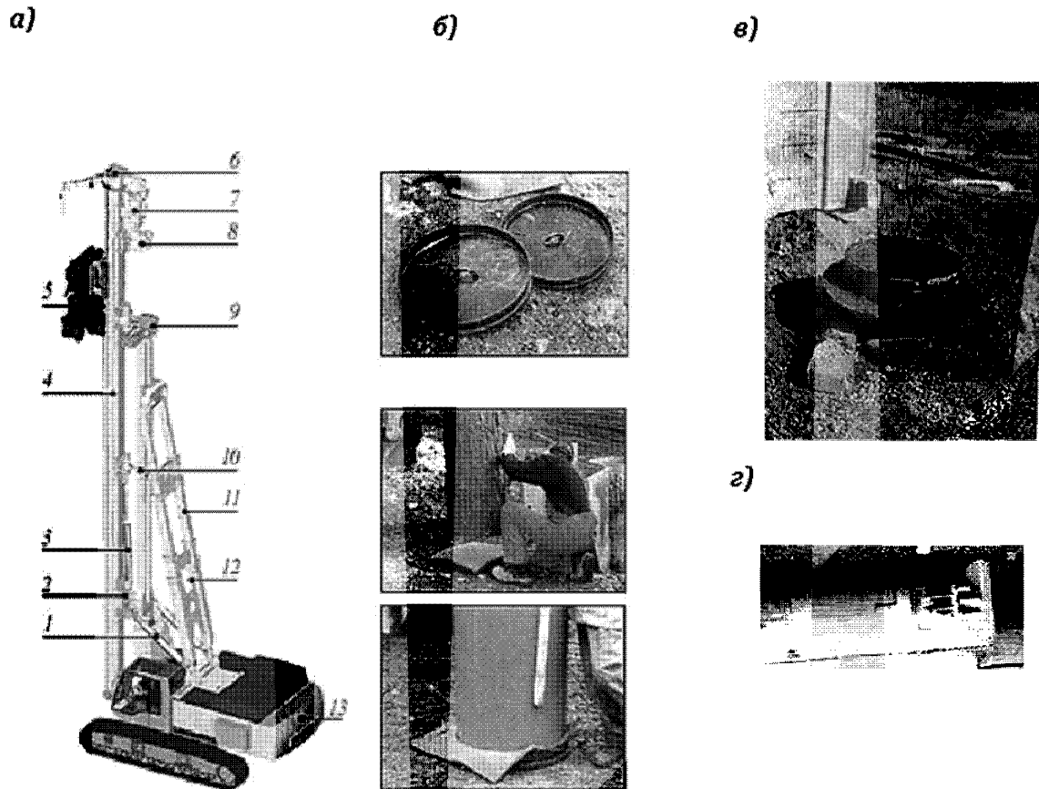
Рис. 8.18. Оборудование для осуществления технологии с вибрационным погружением обсадной трубы:
