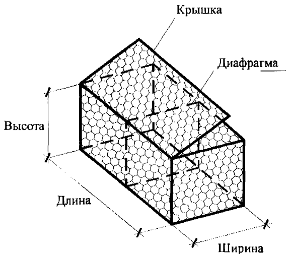
Рисунок 11 – Конструктивная схема габийонных конструкций коробчатой формы
