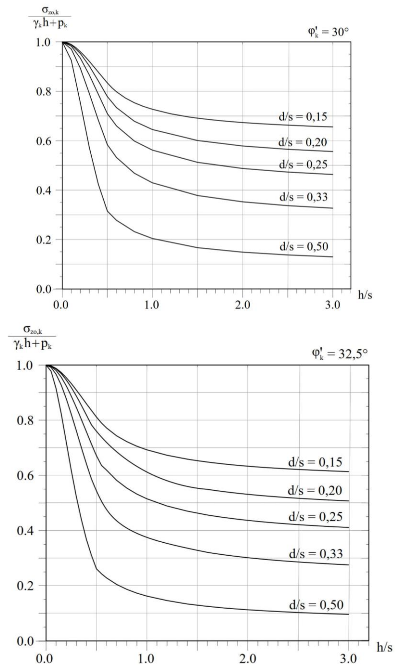
Рисунок А.1 – Графики для проверки мембранных напряжений в армирующем элементе на основаниях из отдельно-стоящих свай ( \varphi'_k = 30^\circ; 32,5^\circ )
