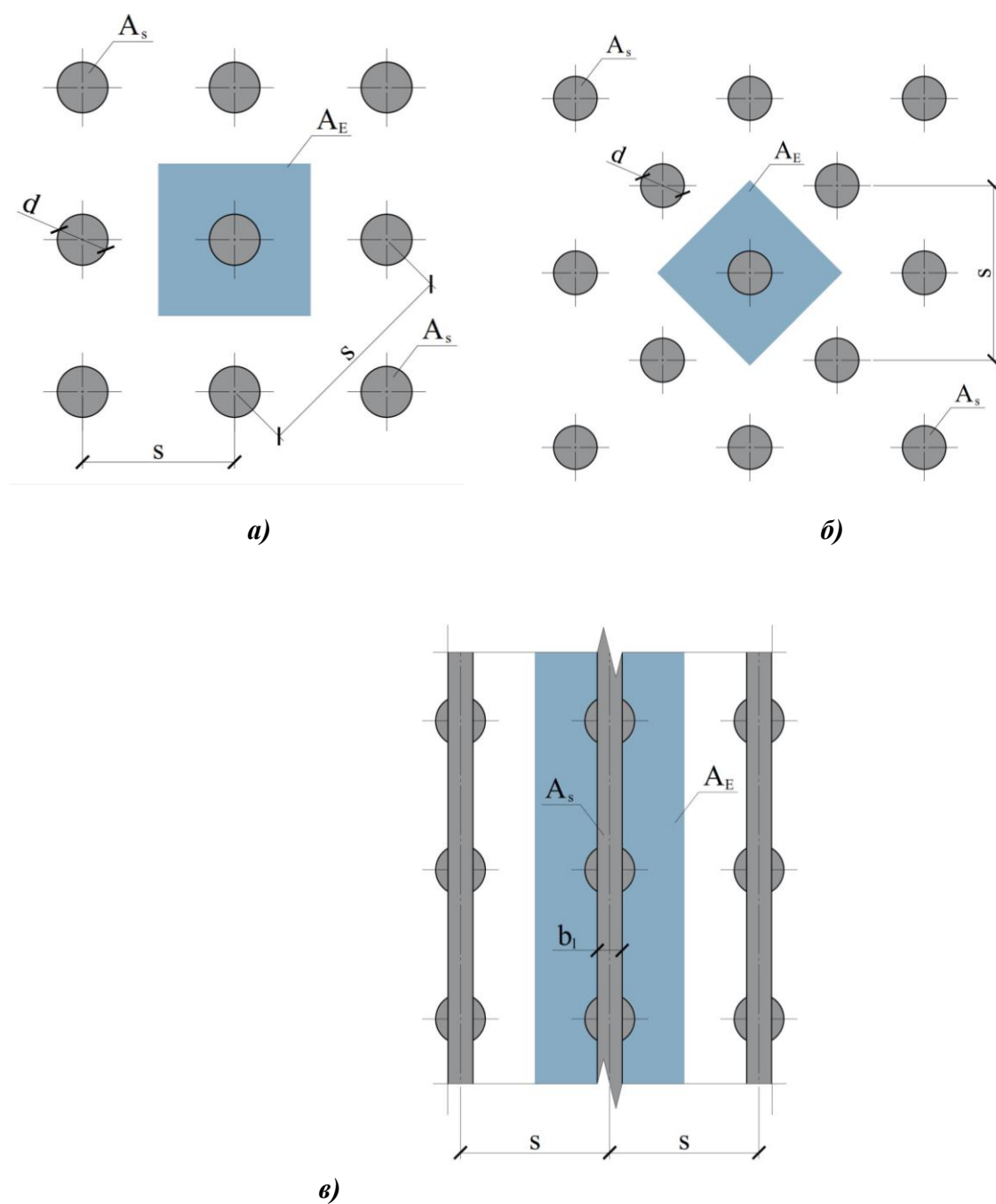
Рисунок 3 – Схемы свайных оснований
