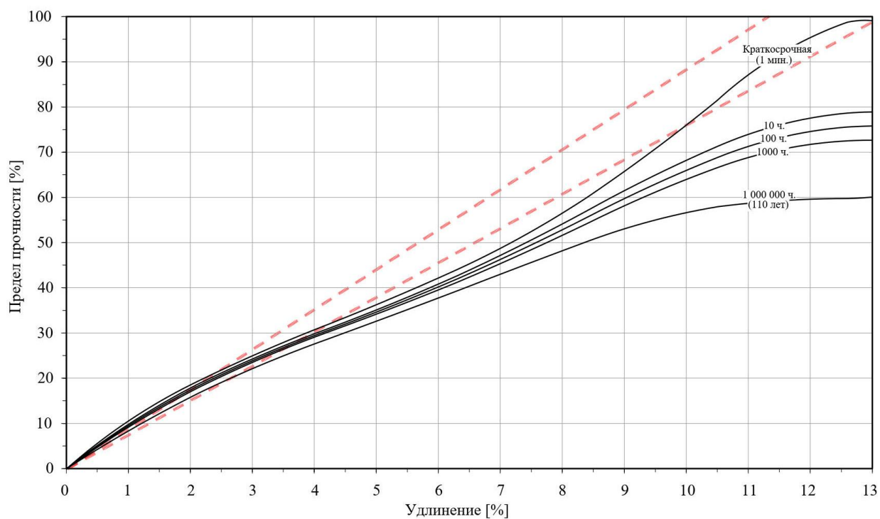
Рисунок Б.2 - Диаграмма деформирования армирующего элемента
