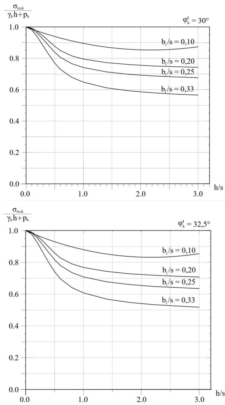
Рисунок А.3 – Графики для проверки мембранных напряжений в армирующем элементе на свайных основаниях с балочным ростверком ( \varphi'_k = 30^\circ; 32,5^\circ )
