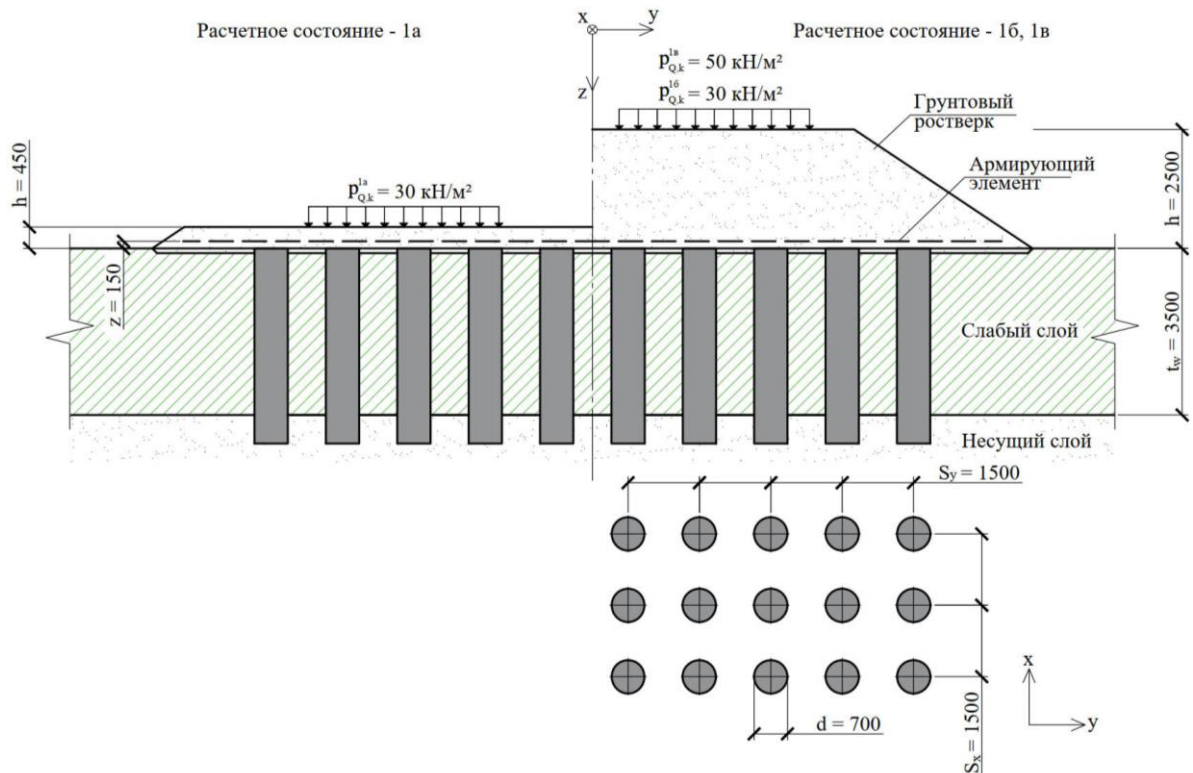
Рисунок В.1 – Расчетная схема
