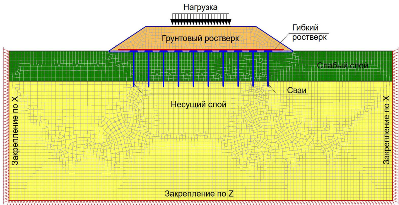
Рисунок Б.1 – Конечно-элементная расчетная модель
