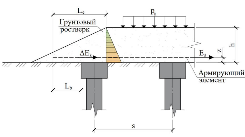
Рисунок 9 – Расчетная схема к определению усилия в армирующем элементе и длины анкерования
