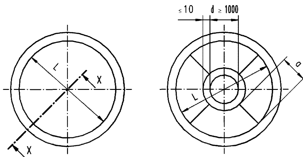
Рисунок 4. Разделение листа антифрикционной пластины (размеры в мм)
