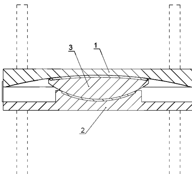
1 – верхняя плита со сферической поверхностью скольжения; 2 – нижняя плита; 3 – скользящий сферический сегмент
