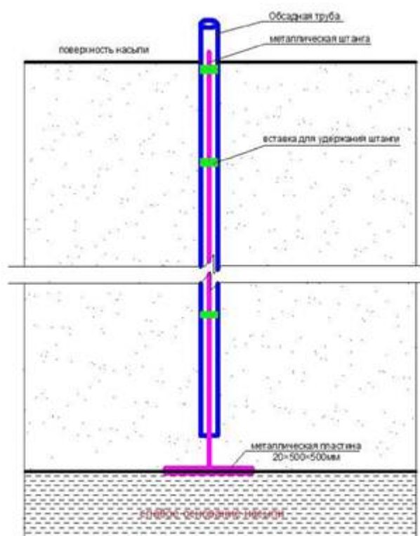
Рисунок 1 - Осадочная марка
