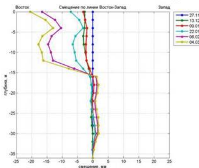
Рисунок 11 - Результаты измерения сползания склона по оси запад-восток
