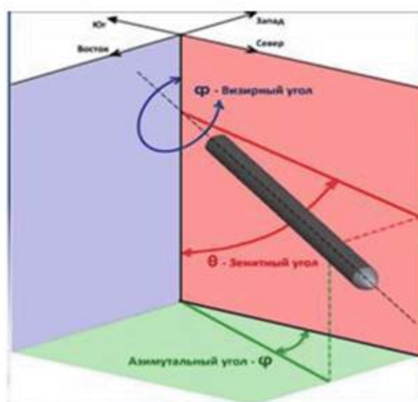
Рисунок 3 - Принципиальная схема инклинометрических измерений при бурении скважин
