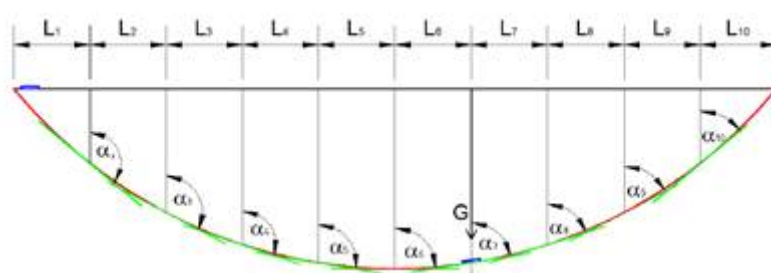
Рисунок 12 - Схема измерения осадок насыпи инклинометром
