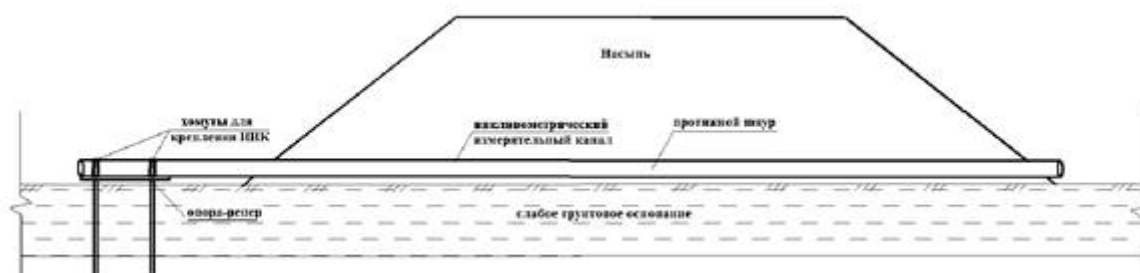
Рисунок 15 - Оборудование измерительного канала
