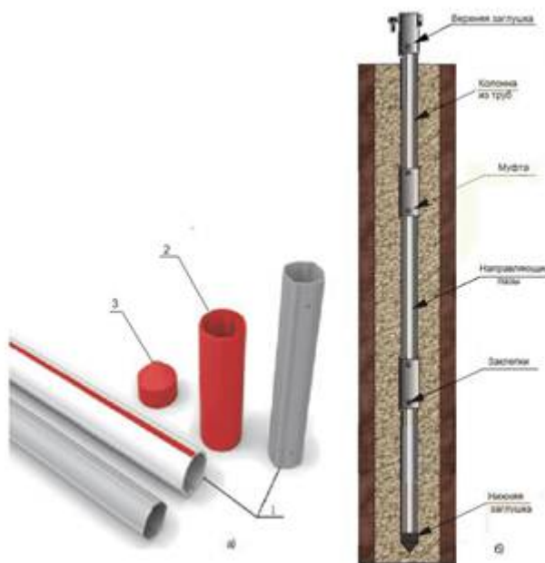
а) 1 - труба, 2 - соединительная муфта, 3 - заглушка б) колонна в сборе
