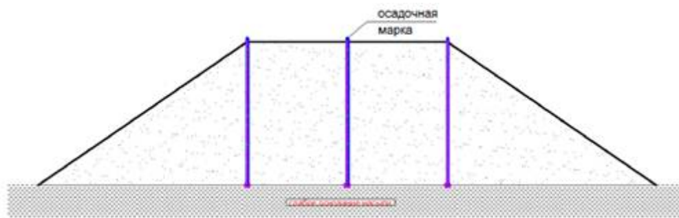
Рисунок 2 - Расстановка осадочных марок для снятия одного поперечника
